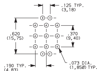
E301J1_BE2 3PDT
