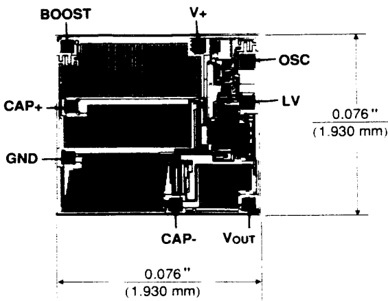
MAX1044
