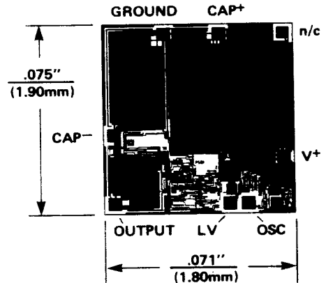
ICL7660
