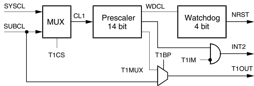
Figure 28. Timer 1 Module
