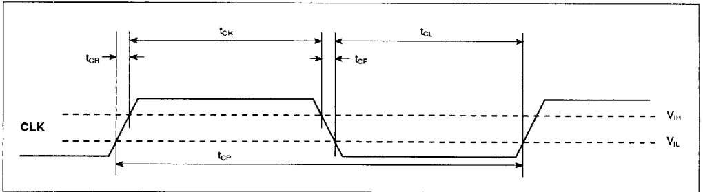
Fig. 5 Clock timing parameters
