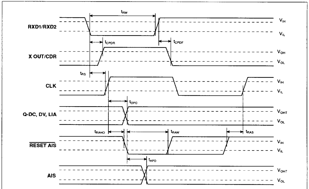
Fig. 6 HDB3 Decoder timing parameters
