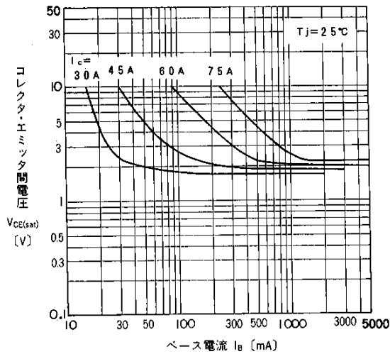
出力特性
