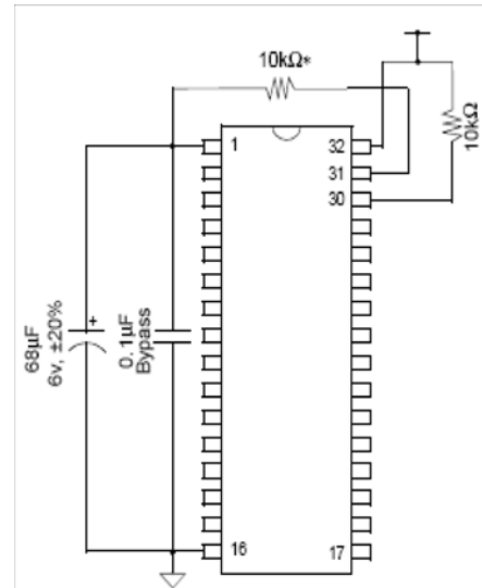
Figure 1. AutoStore® Mode
