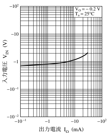
V_{IN} - I_O
