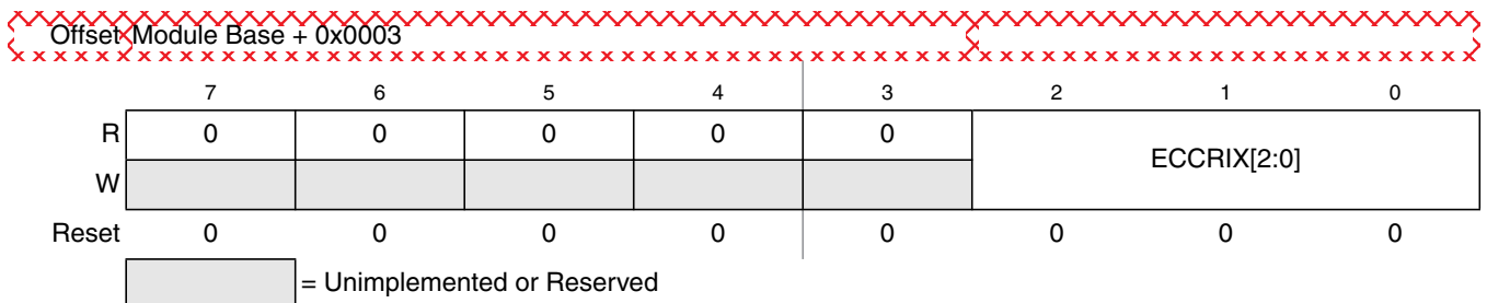
Figure 26-8. FECCR Index Register (FECCRIX)
