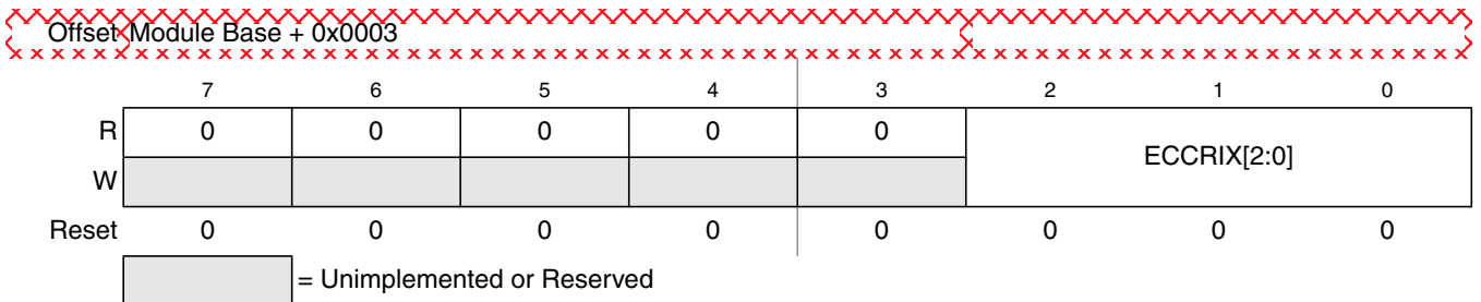
Figure 29-8. FECCR Index Register (FECCRIX)
