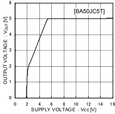
Fig.2 Input Stability(Io=0mA)
