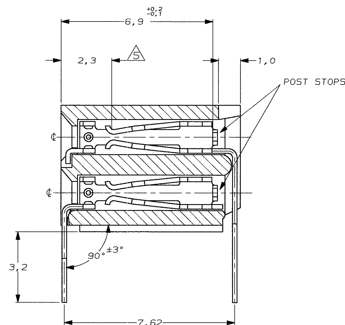
SECTION A-A
