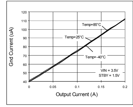
Fig. 71 IOU - IGND
