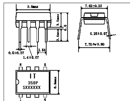
DIP-8
