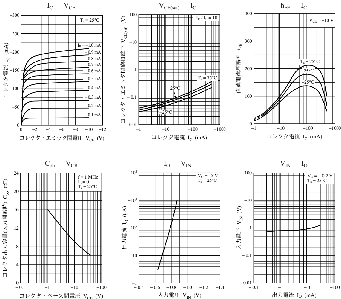
UNR2124 特性図
