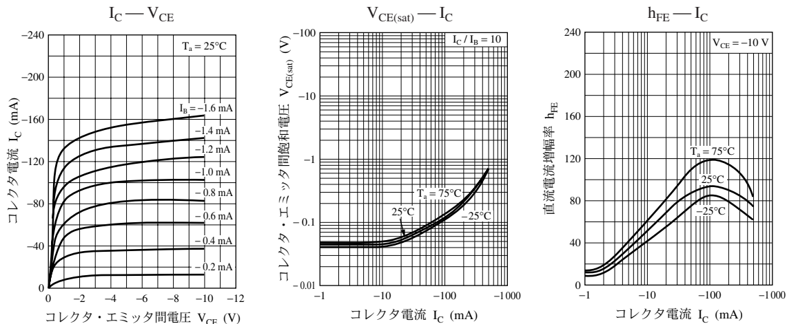
UNR212X 特性図
