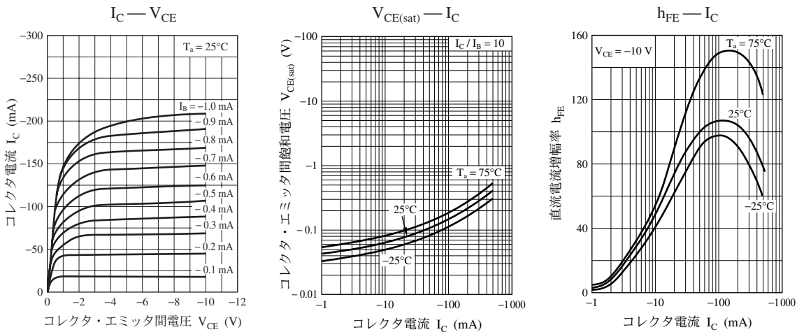
UNR2122 特性図
