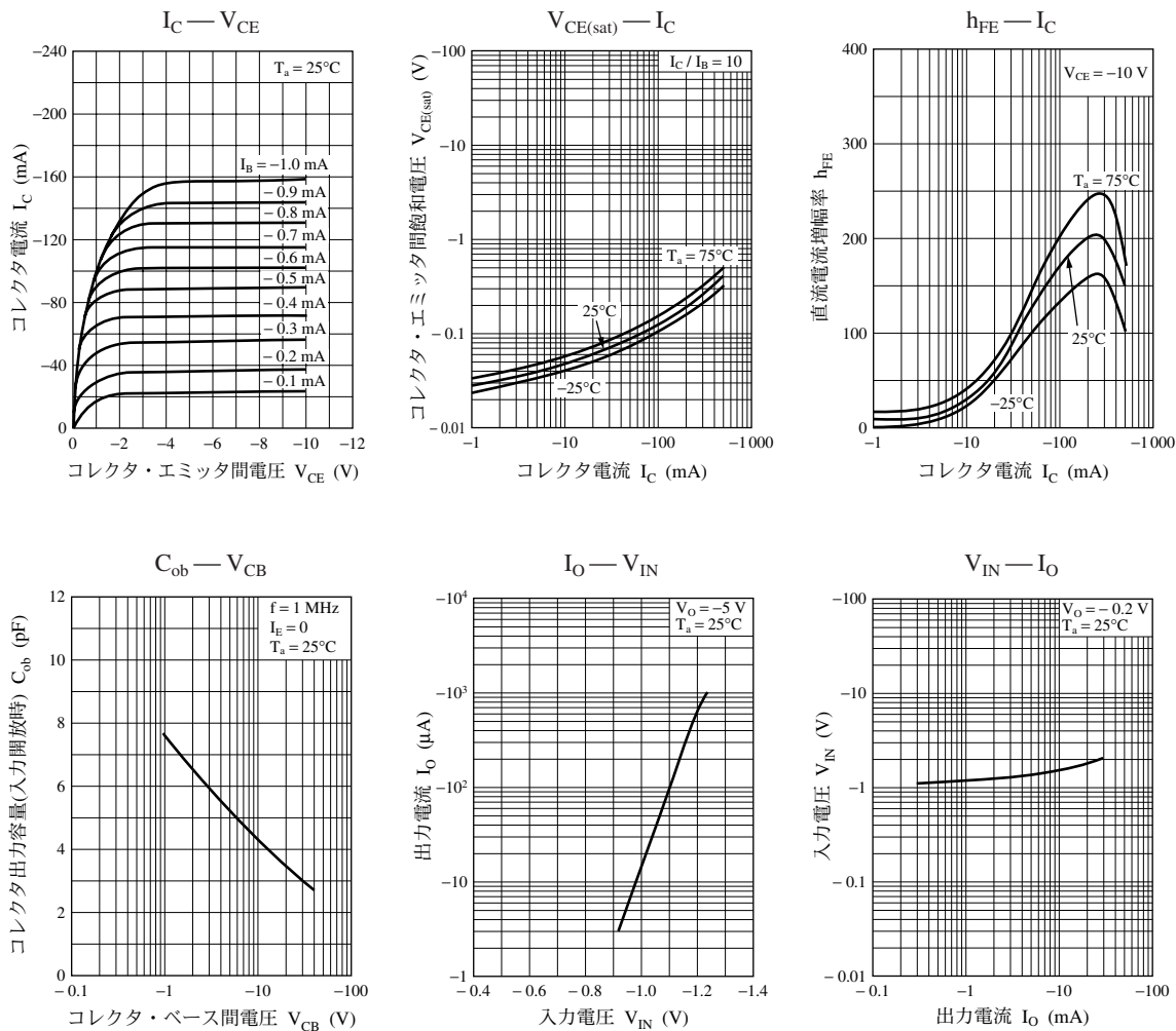
UNR2121 特性図
