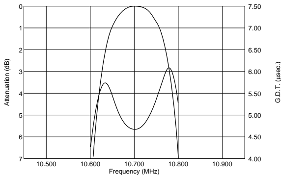
SFELA10M7JAA0-B0
