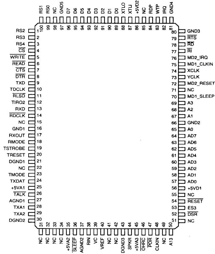
a. 100-Pin PQFP (MD1)
