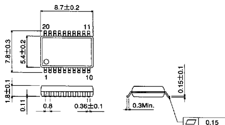
SSOP - A20
