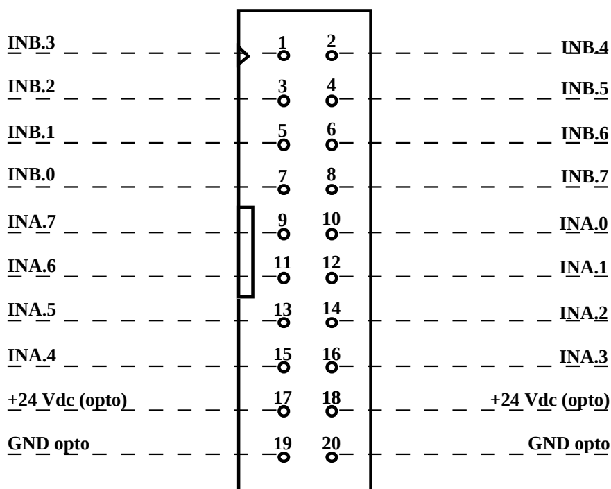
FIGURA 4: K2 - CONNETTORE PER INGRESSI OPTOISOLATI SEZIONI A E B
