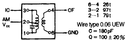
Figure 32 T 2 : AM IFT (455 kHz) 2150-2173-157 (SUMIDA)
