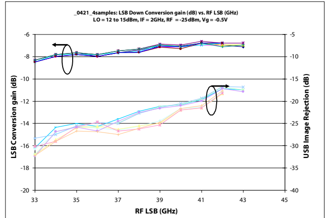
IF=2 GHz
