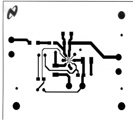
Inner Layer V_{DD}
