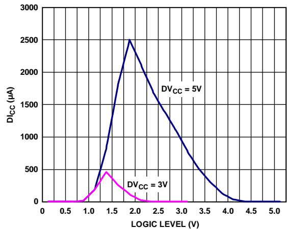
Figure 46. DI CC vs. Logic Input Voltage
