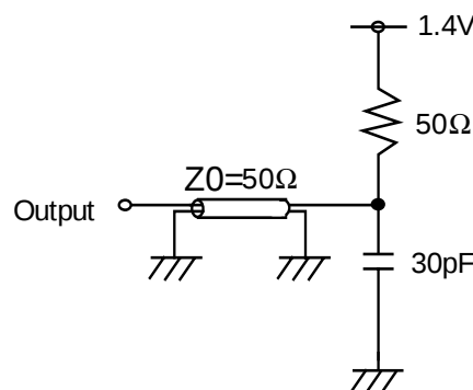
LVTTTL A.C. Test Load (B)
