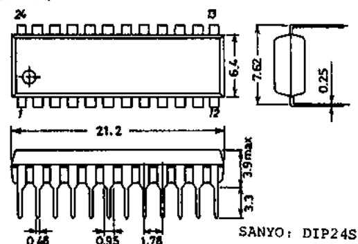
外形図 3067-D24SIC (unit: mm)
