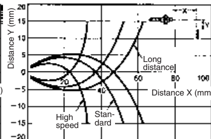
E32-CC200 (Reflective)
