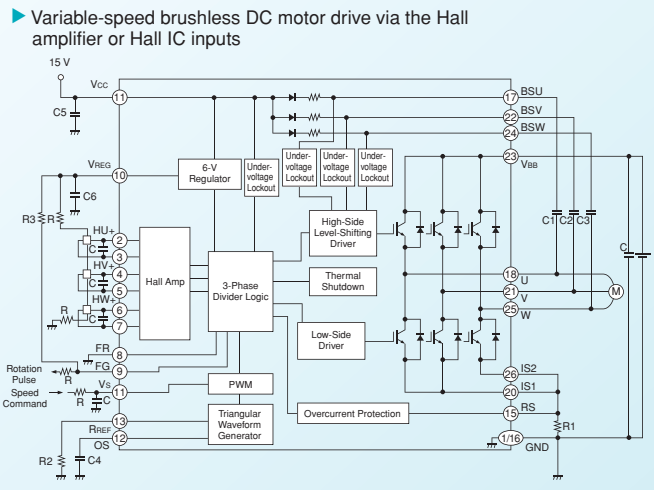
<TPD4121K/TPD4122K Block Diagram>
