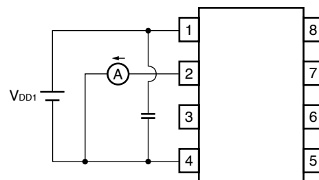
Fig. 4 I_{IL}
