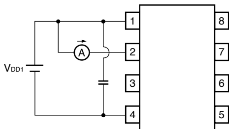
Fig. 3 I_{IH}
