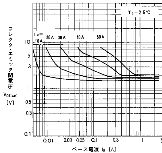
出力特性
