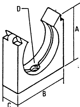
CONDUIT CLIP MATERIAL: NYLON 6
