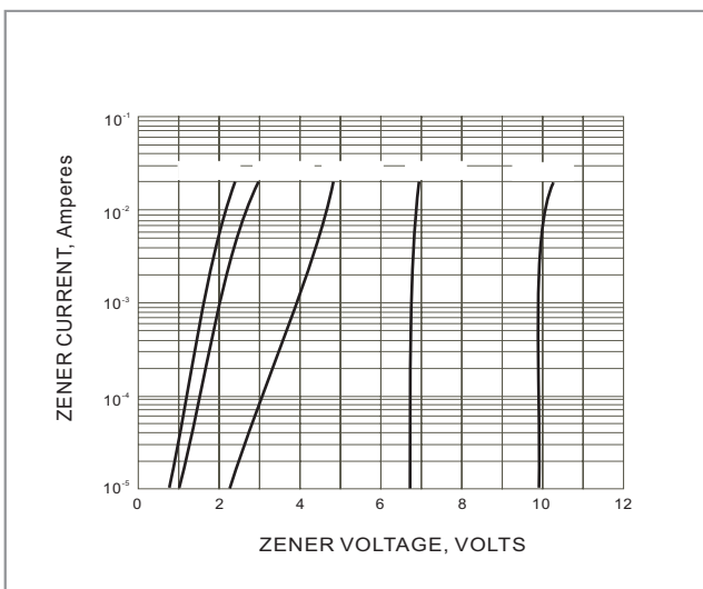
Fig.7 ZENER VOLTAGE VERSUS ZENER CURRENT
