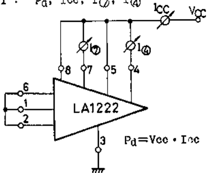
測定回路 1 : P_d, I_{cc}, I_{Q1}, I_{Q2}
