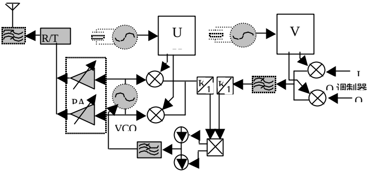
发射机组成框图
