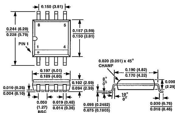
SOIC (R) Package
