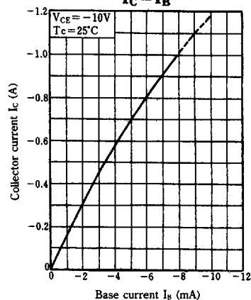
I_C - I_B
