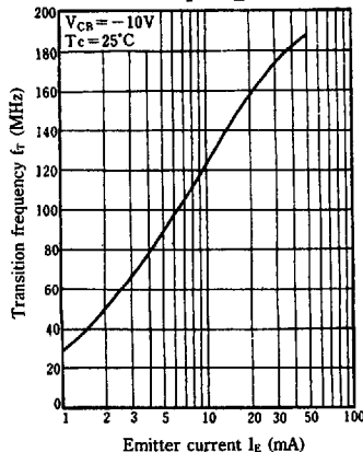
f_T - I_E
