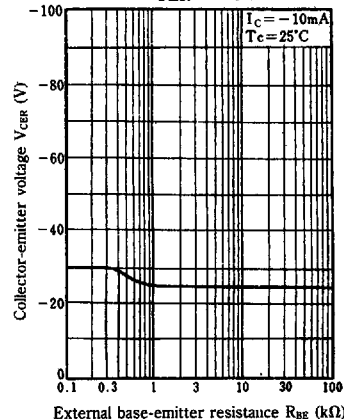
V_{CE} - R_{BE}
