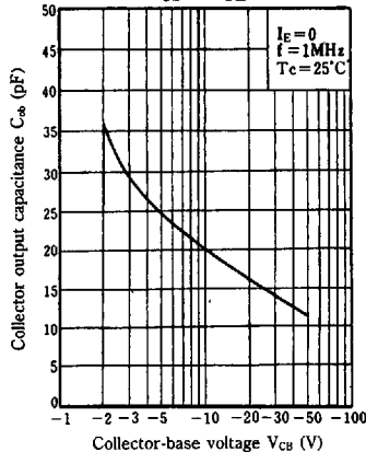
C_{ob} - V_{CB}
