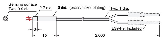
E32-D22L R10
