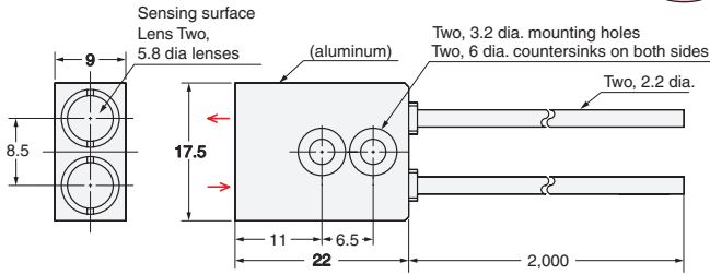
E32-D21L R10
