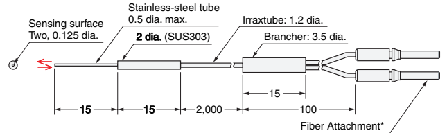
E32-D331 R4
