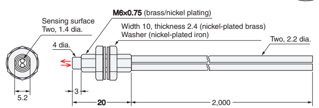
E32-D11L R25
