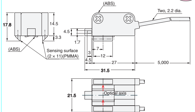
E32-A02 (R4)
