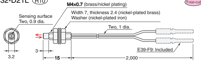
E32-D21L R10
