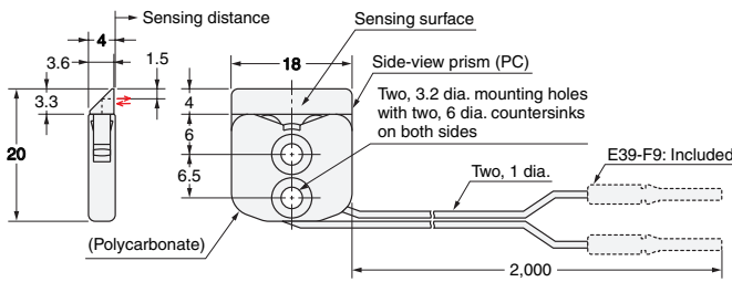
E32-L25 R25
