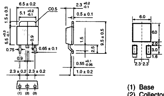
2SD2118F5 (CPT F5)
