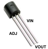
TO-92 (N3)
