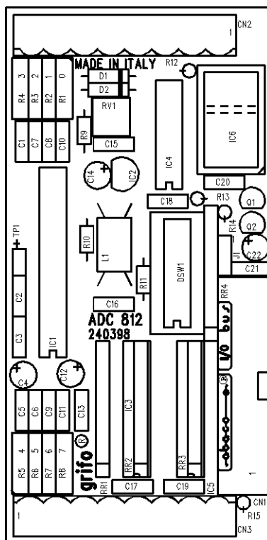
FIGURA 2: PIANTE COMPONENTI
