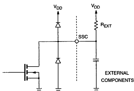
Fig. 2 Pin 11 SSC
