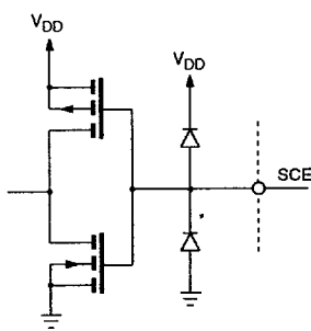
Fig. 3 Pin 14 SCE
