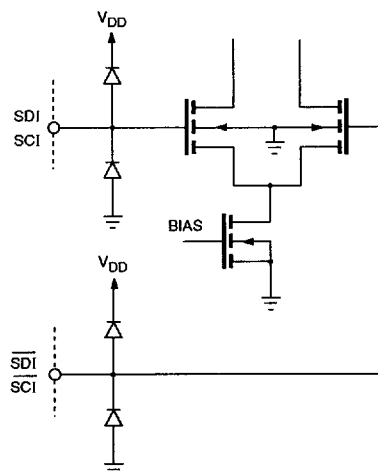
Fig. 4 Pins 5 - 8 SDI - SCI
