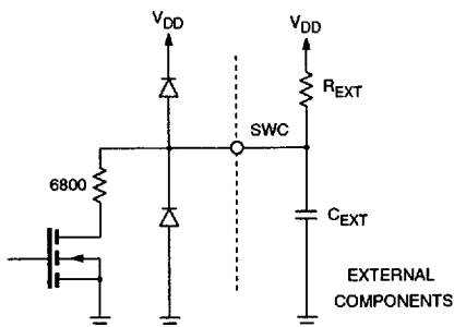
Fig. 5 Pin 15 SWC
