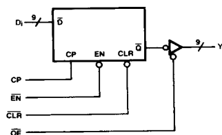
Am29824A
