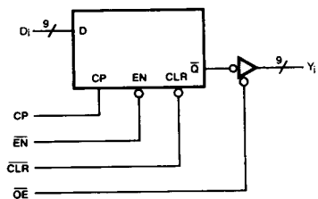
Am29823A
