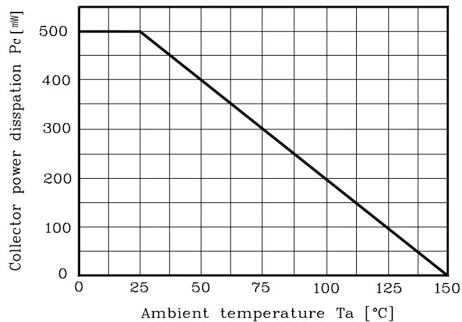
Fig. 1 P_C - T_a
