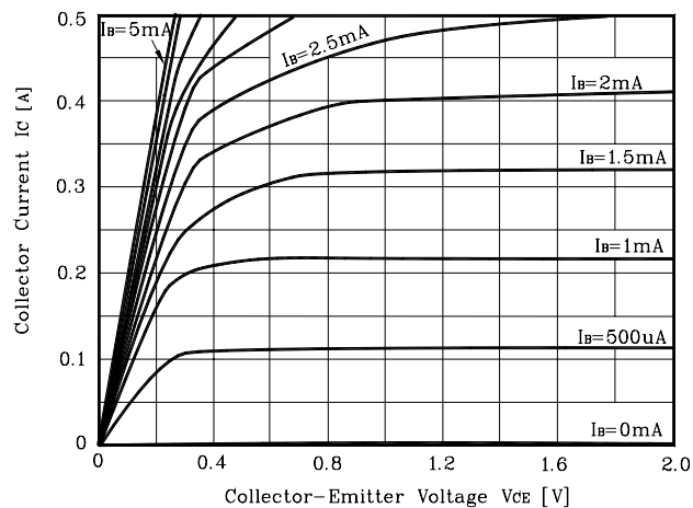
Fig. 4 I_C - V_{CE}
