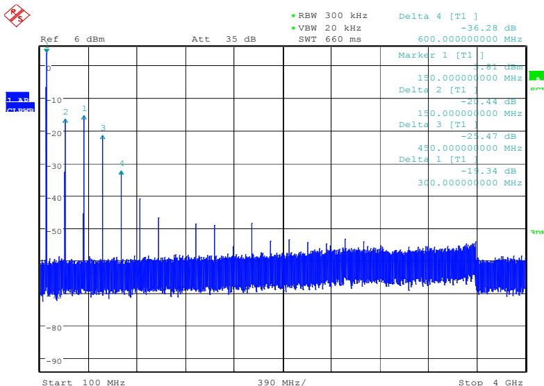
Harmonic suppression
