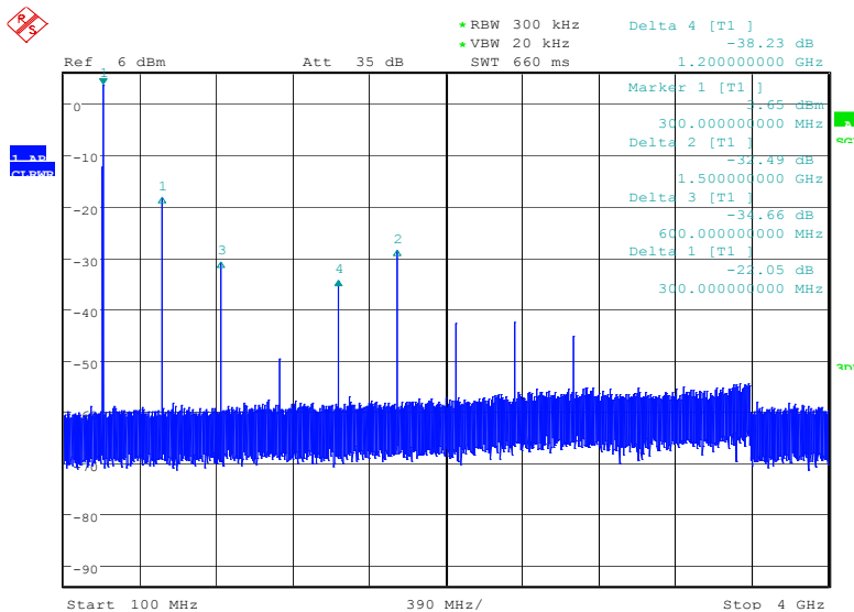
Harmonic suppression
