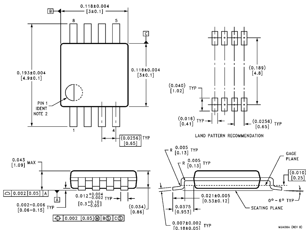
Surface Mount Mini SO-8 Package NS Package Number MUA08A
