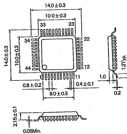
QFP 44pin
