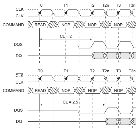
FIG. 4 CAS LATENCY
