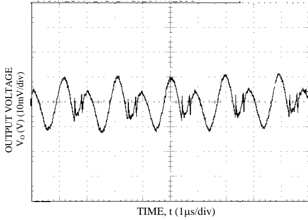
V_o=0.7V , T_a=25^\circ C , V_{in}=12V , I_o = I_{o,max}
