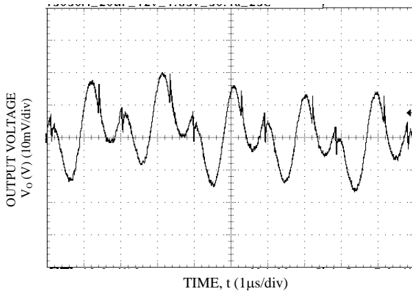
V_o=1.8V , T_a=25^\circ C , V_{in}=12V , I_o = I_{o,max}
