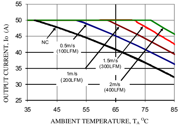
V_o=0.7V , V_{in}=12V
