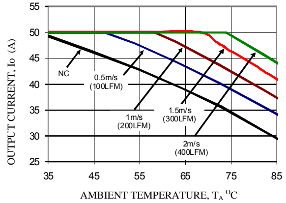
V_o=1.2V , V_{in}=12V
