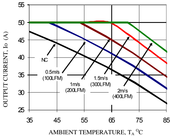
V_o=1.8V , V_{in}=12V
