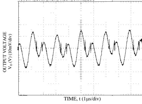
V_o=1.2V , T_a=25^\circ C , V_{in}=12V , I_o = I_{o,max}
