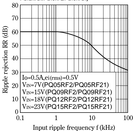
Fig.23 Ripple Rejection vs. Input Ripple Frequency (PQ05RF2/PQ05RF21/PQ09RF2/PQ09RF21/PQ12RF2/PQ12RF21/PQ15RF2/PQ15RF21)
