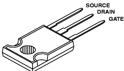
JEDEC TO-220AB
