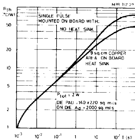
Figure 28 : SO (12 + 4 + 4).
