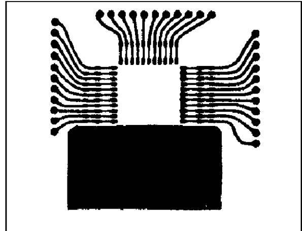
Figure 29 : PLCC (33 + 11).
