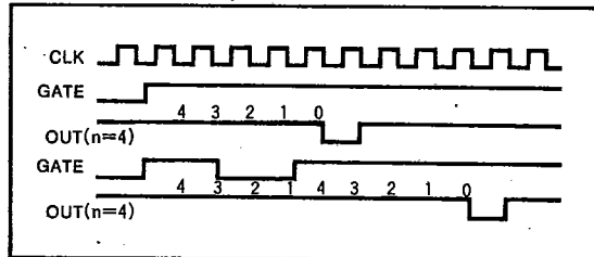
Fig. 7 Mode 5
