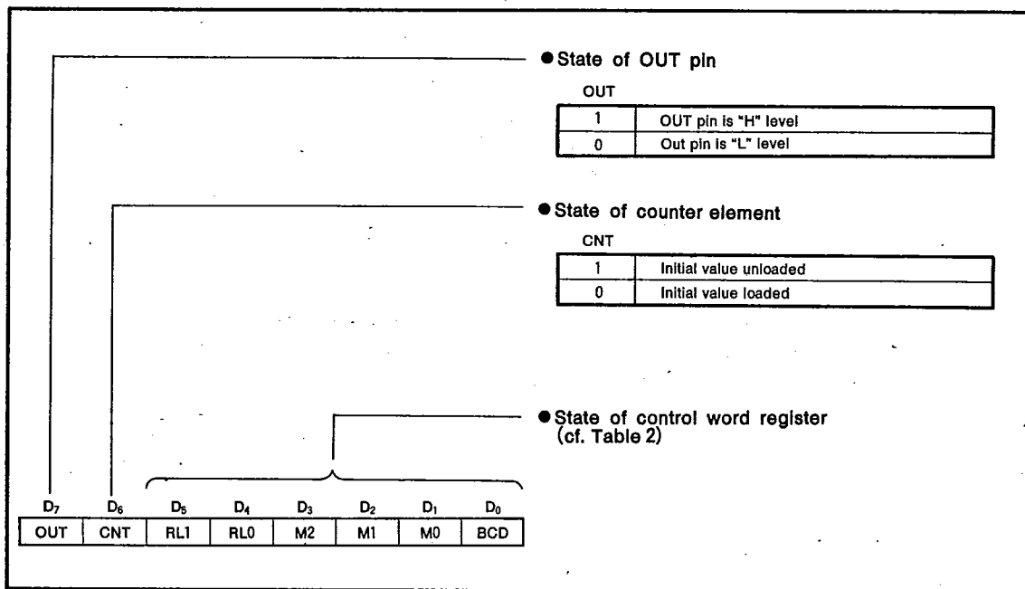
Fig. 9 Status Byte
