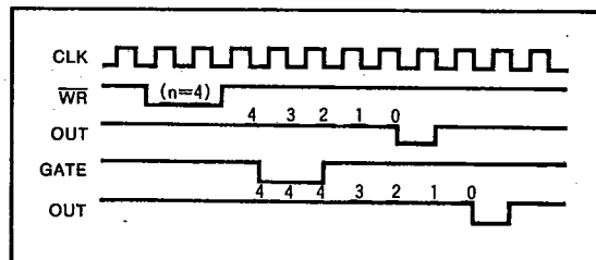
Fig. 6 Mode 4
