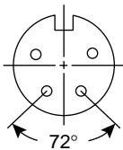
4 Pin 164-6040
